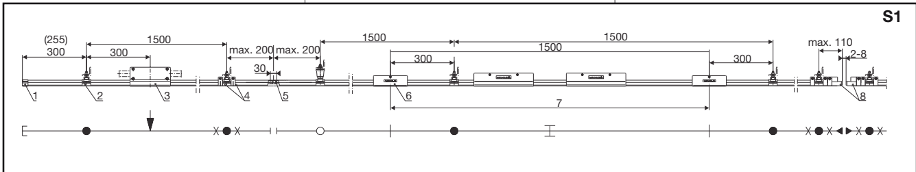
Verlegungsplan
